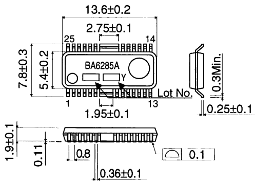
HSOP25 (Unit:mm)
